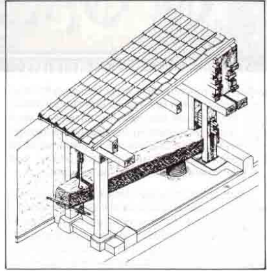
Bulunan yapılar arasında, Akdeniz Bölgesi'nde görülen zeytin presleri de vardır. Bu eski preslerin kalıntılarında Provence'ta sıklıkla rastlanmıştır. Burada, Var'daki Taradeau'da bulunan bir presin rekonstrüksiyonu görülmüyor (J.P. Brun'e göre).
