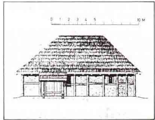
Bütün villalar büyük ve taştan yapılmış değildi, çoğu kerpiç ve tahtadan inşa edilmişti. Meselâ İsviçre'deki Laufen-Müschenberg'te bulunan bu villanın rekonstrüksiyonunda aynı duruma rastlanıyor (Daunier'ye göre).
