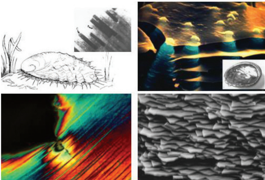
Sedef. Kaliforniya kıyılarında yaşayan bu deniz kabuklusunun ( Halotis rufescens , solda üstte) içi sedeften; kalsiyum karbonat ve protein katmanlarından oluşuyor. Bu tuğla ve harç bileşenli yapı mühendislerce bilinen sert ve güçlü yapı. Bu materyal, sol üstte taramalı elektron mikroskobu (SEM) ile elde edilen görüntüde olduğu gibi bilim adamlarının "self-assembly" dedikleri bir şekilde formunu alıyor. Bu yapısal özellikler bu canlıların neden bu kadar uzun süre hayatta kalabildiklerini açıklıyor. (550 milyon yıldır!) Bilim adamları ve mühendisler bu yapılardan öğrendiklerini günlük kullanılacak biyomimetik materyallerin yapımında kullanacaklar.
