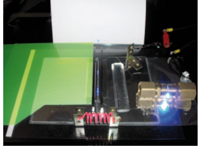
Hava lazeri çalışırken. Kıvılcım anahtarı ve plazma kanalı ışıltıyor. Karşıdaki beyaz kağıt üzerinde lazer ışını parıltması görünüyor. Soldaki sarı plastik parça, elektrot açısı ve aralığını güvenle ayarlamak için kullanılıyor.
