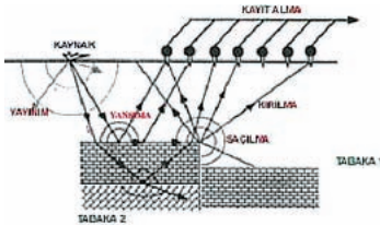
Şekil 2. Dalga Yayılım Diyagramı.
